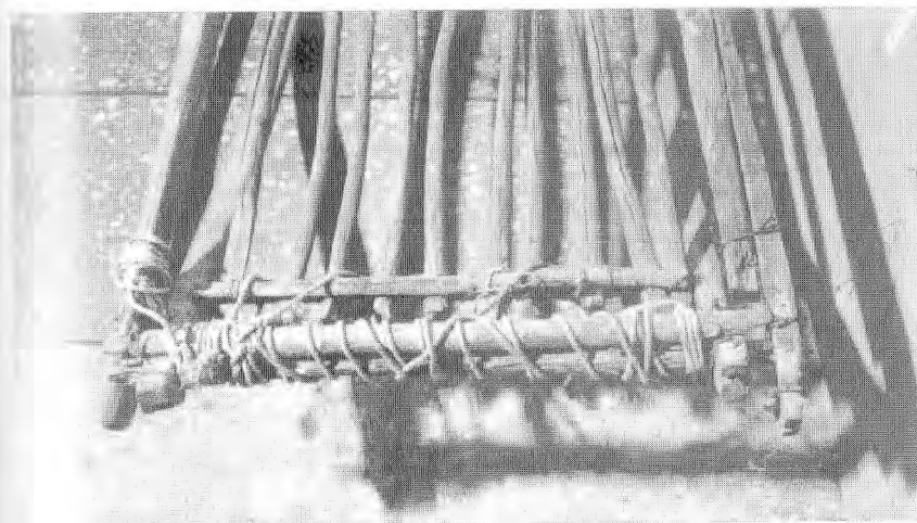
Рис. 71. Охотничья нарта токи (нанайцы, кол. КМКМ).
