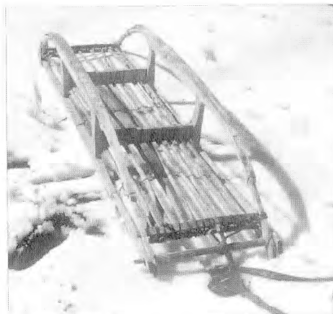
Рис. 75. Охотничья нарта токи (нанайцы, с. Джари). Фото автора, 2001 г.
