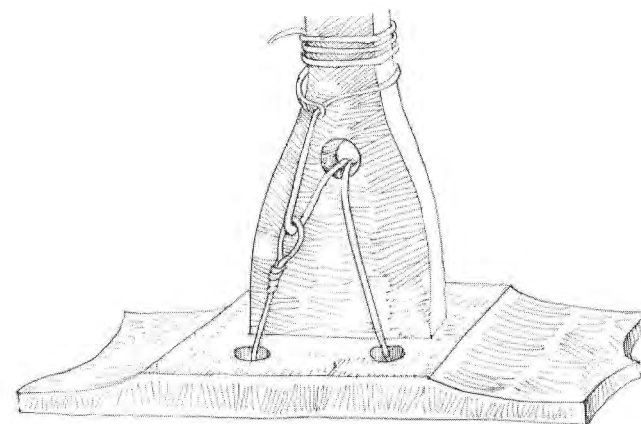
Рис. 83. Восточносибирские нарты пара и крепление копыла (полосом) (по ИЭА).
