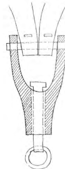
Рис. 108. Конструкция вертлюгов: махтыгень (удэгейцы, дерево), махт (нивхи, бронза).
