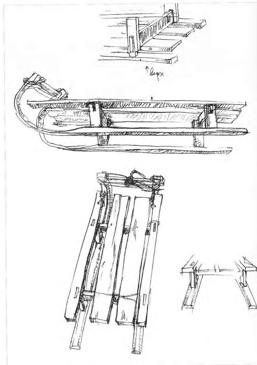
Рис. 88. Санки парака (ПМА 1996 г., с. Найхин).
