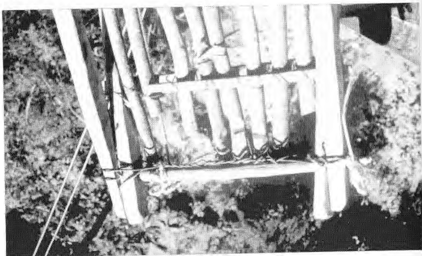
Рис. 69. Фрагменты охотничьей нарты токи (нанайцы, Улика-Национальное, р. Кур). Фото автора, 2004 г.
